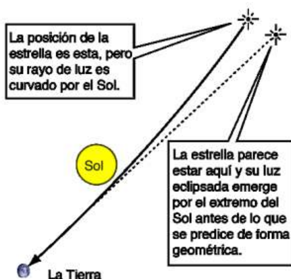
Figura 2. Deflexión de la luz de un estrella por presencia del Sol.
