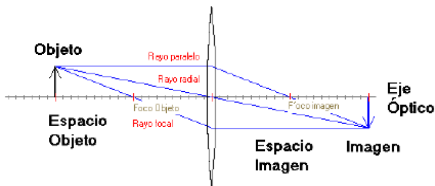
Figura 8. Óptica Geométrica. Marcha de rayos.
