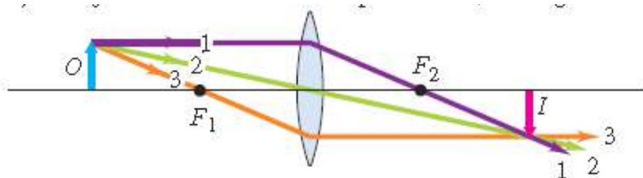
Fig. 9 Objeto más alejado de la lente que el foco. a) Objeto muy alejado del punto Focal, b) Objeto más cerca del punto focal
