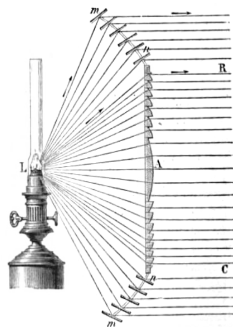
Figura 2. Lente de Fresnel: marcha de rayos
