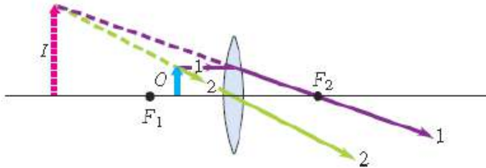
Fig 10. El Objeto esta más cerca de la lente que el foco. La imagen es virtual, derecha y más grande que el objeto.
